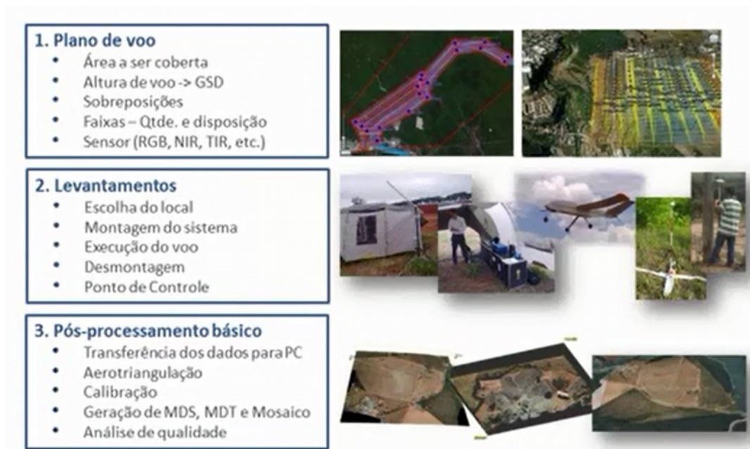
Figura 23: Etapas da Fotogrametria/Topografia aérea
