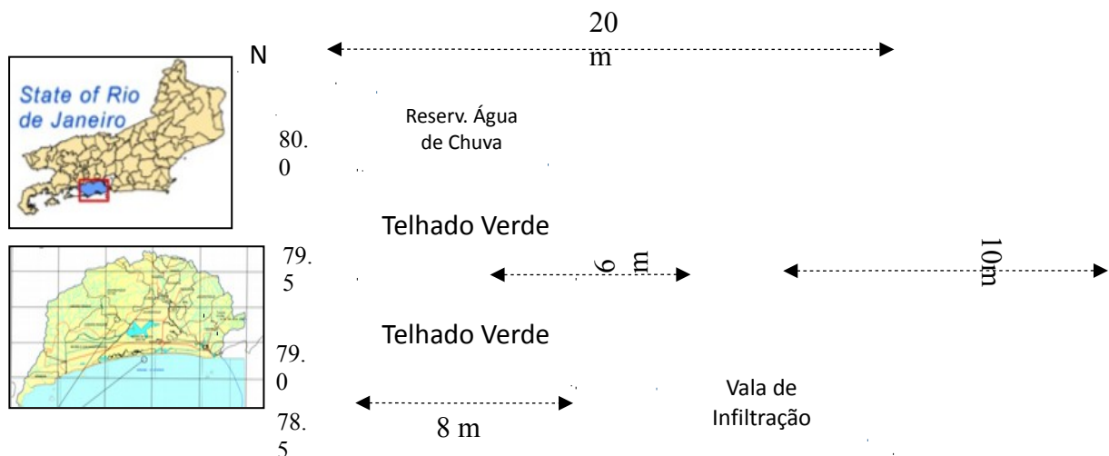
Figura 2: Área de implantação de técnicas compensatórias de drenagem urbana em lote residencial no bairro da Tijuca, RJ.
